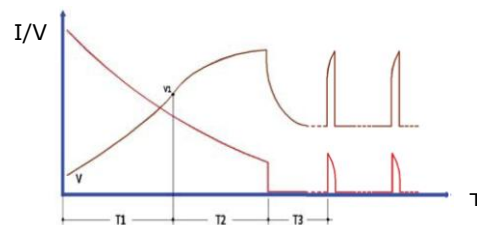
Стандартный цикл заряда
