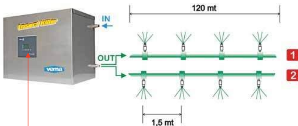
Программируемый ПЛК
