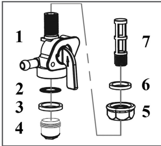
Рис. 19 Устройство топливного крана
