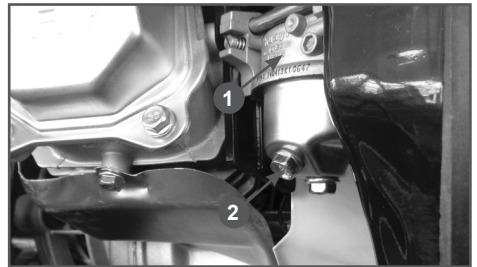
Рис. 20 Слив топлива из карбюратора
